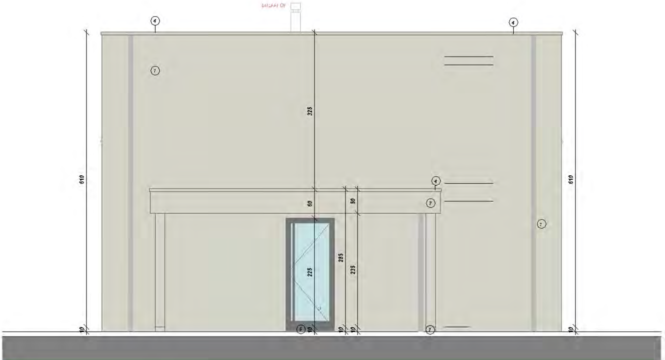
RECHTER ZIJGEVEL LOT 18
