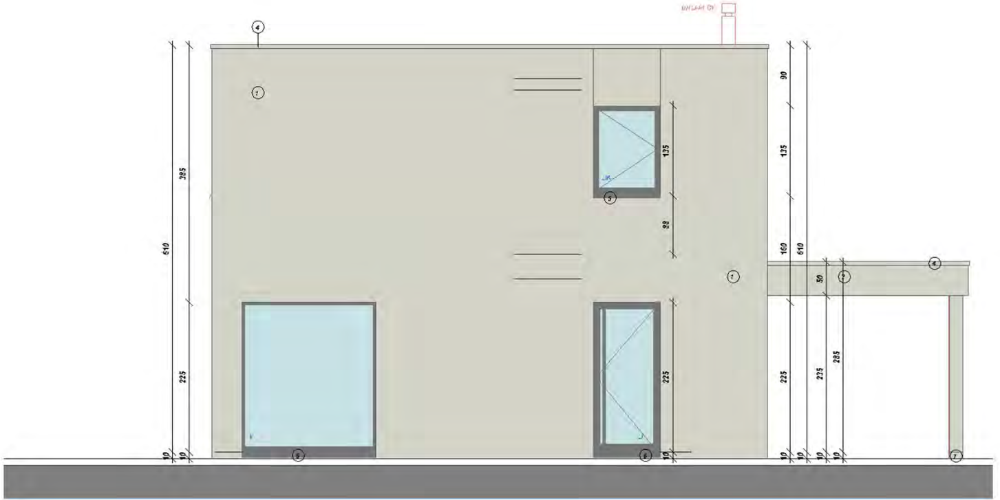
VOORGEVEL
