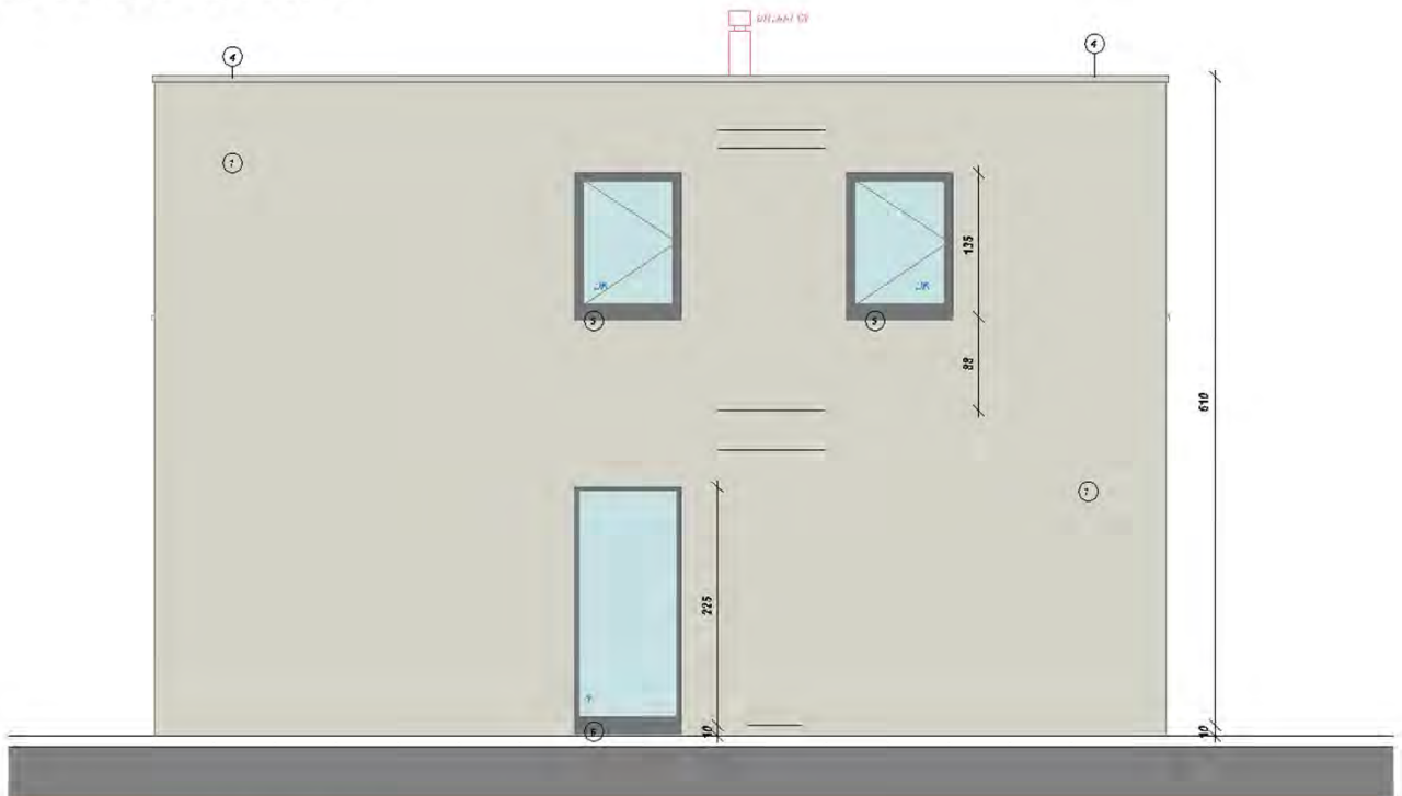
RECHTER ZIJGEVEL LOT 18
